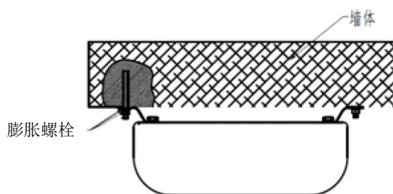
安装示意图
