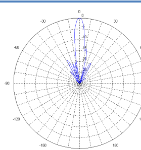
820-960/1710-2170MHz
