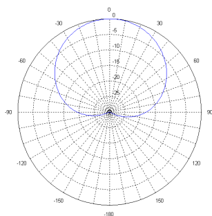
水平面方向图 Horizontal pattern
